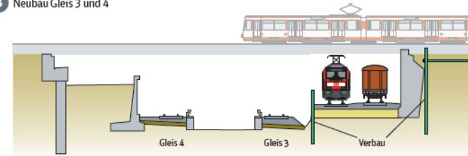
4 Abriss der alten Gleise, Neubau Widerlager und Pfeiler
