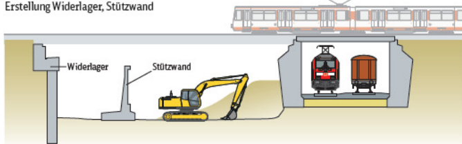
2 Aushub für Streckenneubau, Erstellung Widerlager, Stützwand
