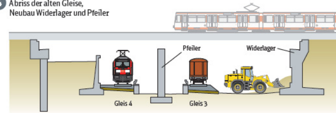
5 Neubau Gleise 1 und 2, Brückenbauwerk
